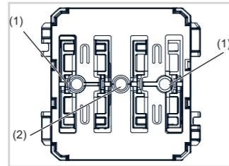
Bild 1: Frontansicht Taster-Modul
